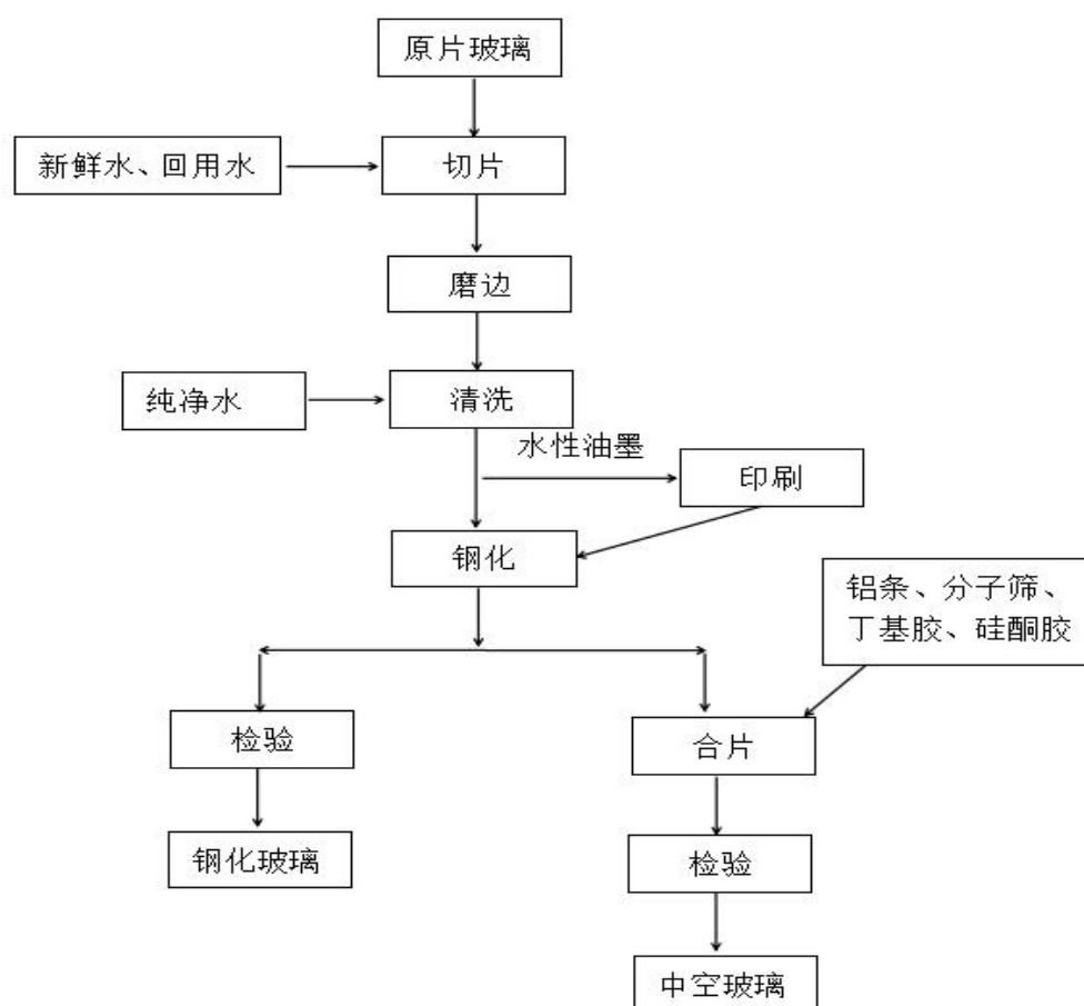
图 1-2 生产工艺及产污环节图
